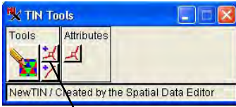
Add Node
